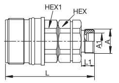
Male Thread 24° cone – DIN 2353
